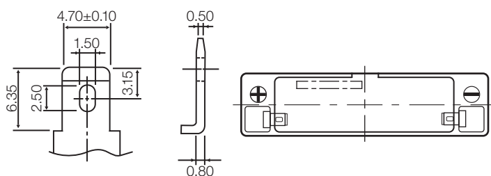
Faston tab : 187 (Standards)
