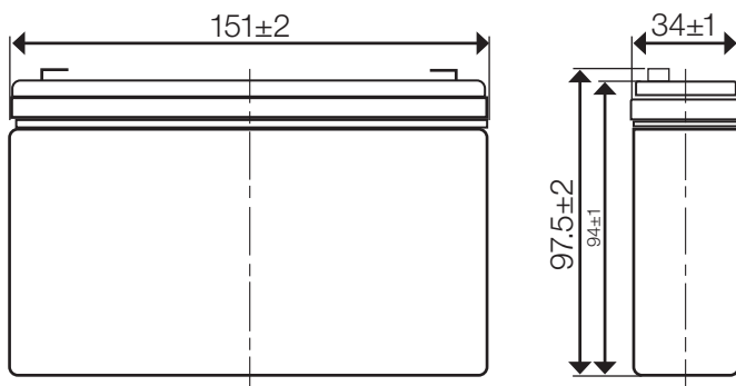
Faston tab : 187 (Standards)
