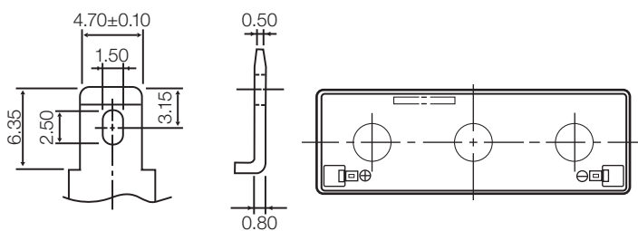
Faston tab : 187 (Standards)
